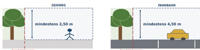
Freizuhaltende Lichtraumprofile
